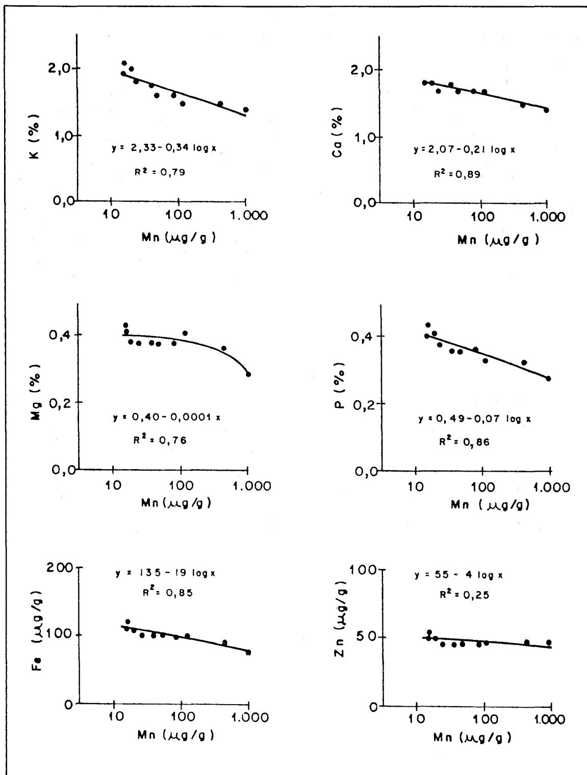
FIGURA 4. Concentración Mn en solución nutritiva vs. nivel foliar de otros minerales, en lentejas. FIGURE 4. Mn concentration in nutritive solution vs. foliar level of other minerals, in lentils.
