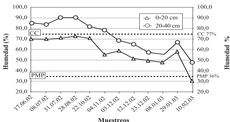
Figura 3. Evolución del contenido de humedad (%) del suelo con trigo. Carillanca, 2002-2003. Figure 3. Evolution of moisture content (%) of soil with wheat. Carillanca, 2002-2003.
