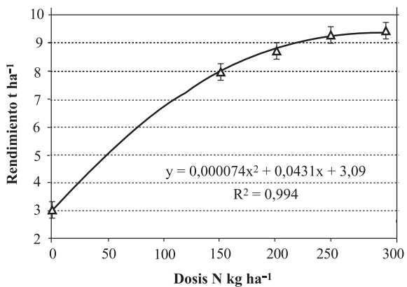
Figura 6. Incremento del rendimiento de trigo según dosis anual de N. Carillanca, 2003-2004.
