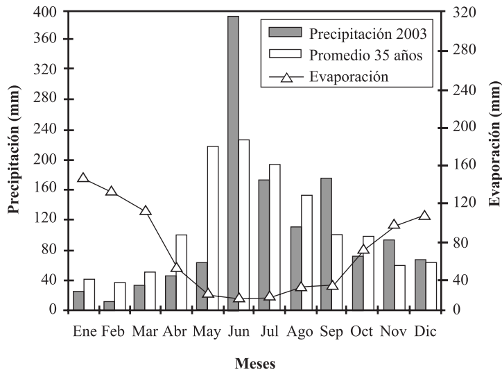
Figura 2. Antecedentes del clima en la localidad Carillanca durante el año 2003. Figure 2. Climatic information of Carillanca locality during year 2003.
