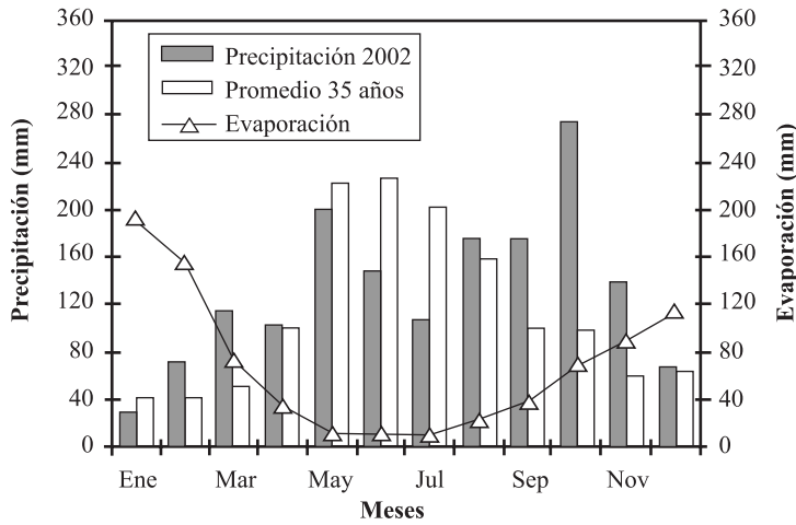
Figura 1. Antecedentes del clima en la localidad Carillanca durante el año 2002. Figure 1. Climatic information of Carillanca locality during year 2002.
