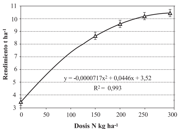
Figura 5. Incremento del rendimiento de trigo según dosis anual de N. Carillanca, 2002-2003.
