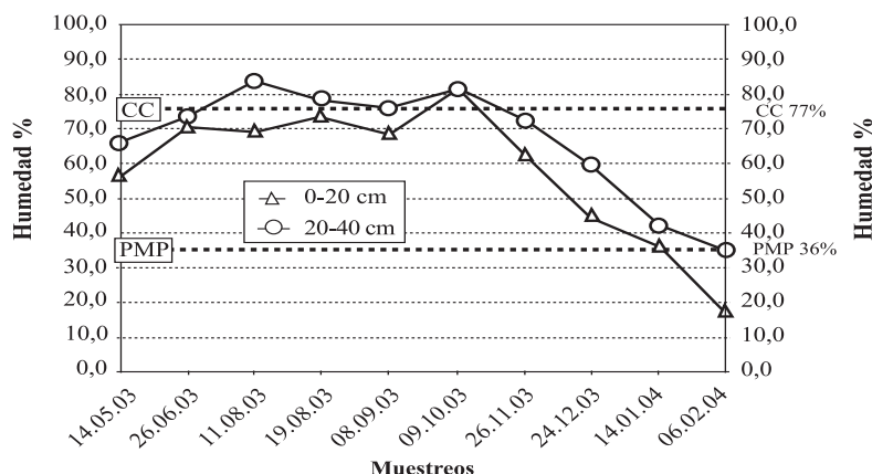
Figura 4. Evolución del contenido de humedad (%) del suelo con trigo. Carillanca, 2003-2004. Figure 4. Evolution of moisture content (%) of soil with wheat. Carillanca, 2003-2004.
