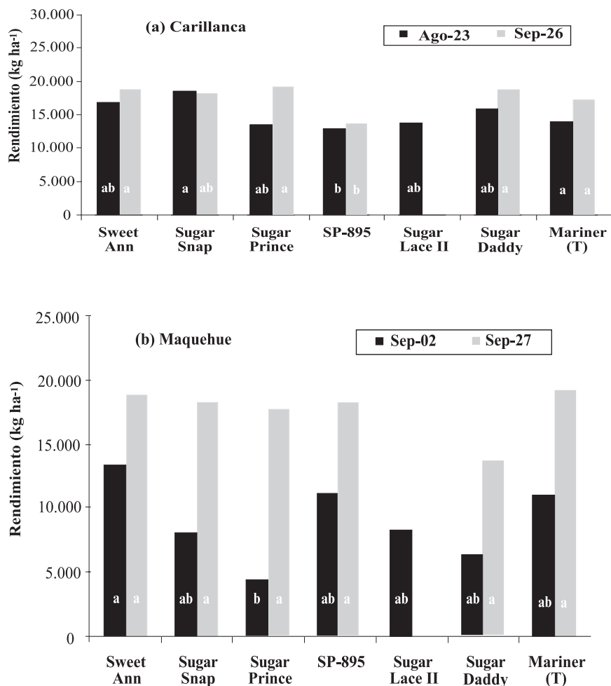
Figura 2. Rendimiento en vaina de variedades de arveja tipo “sugar snap” en dos épocas de siembra, durante 2005. (a) Carillanca, (b) Maquehue.
