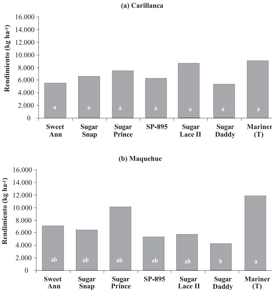
Figura 1. Rendimiento en vaina de variedades de arveja tipo “sugar snap” en dos épocas de siembra, durante 2004. (a) Carillanca, (b) Maquehue.
